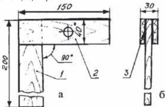
Расми 7. Нақшаи васлии гунё: а – намуди асосӣ; б – намуд аз чап
