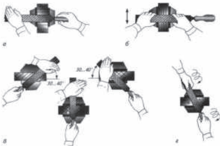
Расми 46. Усули сӯҳонкунии маснуот: а – арзӣ; б – барқадӣ; в – салибмонанд; г – доиравӣ.
