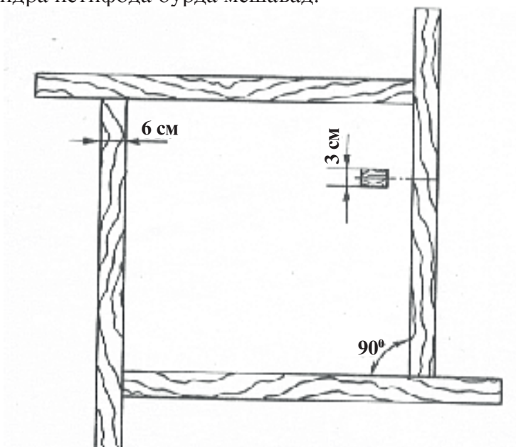
Расми 70. Чорчӯба барои рехтани гач
