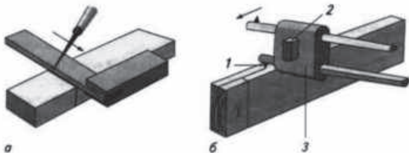
Расми 9. Андозагузори маснуоти пайвастагии зинадори кунҷӣ: а – кўндалангӣ бо гунё; б – барқадӣ бо рейсмус: 1 – поя, 2 – фона, 3 – асос.
