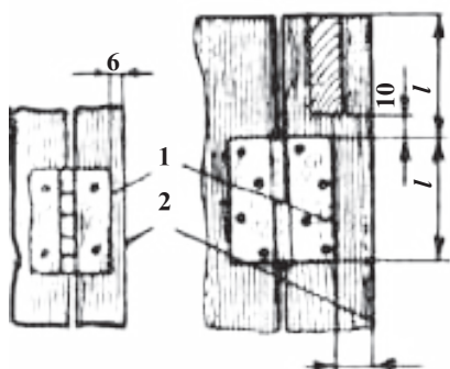
Расми 51. Нақшаи ҷобачокунии ошиқ-маъшуқи бодхон (а) ва тиреза (б): 1-канори барқадӣ; 2-қирраи паҳлуии чортарош.
