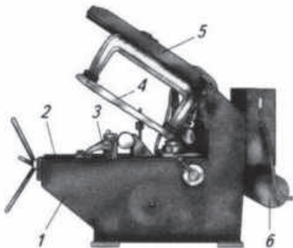
Расми 40. Арраи механикӣ: 1 – асос; 2 – миз; 3 – хартум; 4 – тасмаохан арра; 5 – муҳаррики барқӣ; 6 – гироҳои мошинӣ
