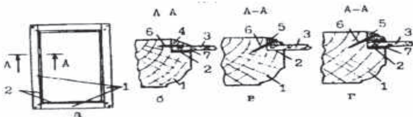
Расми 55. Чорчӯбаи тиреза (а) ва маҳкам кардани шиша бо хамираи дуҷабата (б), бо рейкаҳо (в), бо хамира ва ҷӯбчаҳои чортарош (г): 1 – чорчӯбаи тиреза; 2 – ҷӯякҳо; 3 – шиша; 4 – хамира; 5 – рейкача; 6 – мех; 7 – хамираи зери шиша.
