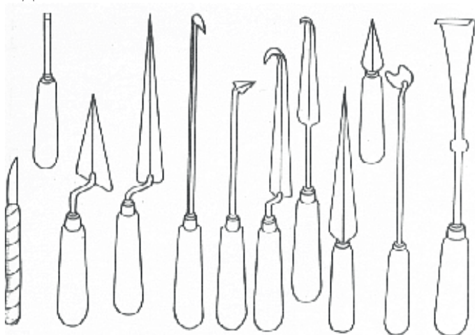
Расми 69. Асбобҳои махсуси гачқорӣ
