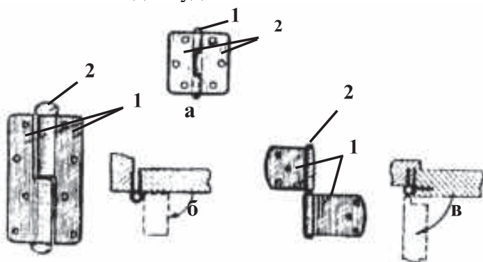
Расми 50. Сохти ошиқ-маъшуқи бодхон (форточка) (а), рӯякӣ (б) ва комакии (в) тиреза: 1-карта; 2-чап-рост.
