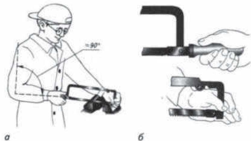
Расми 38. Кор бо дастарра: а – ҳолати корӣ; б – ҳолати дастон.
