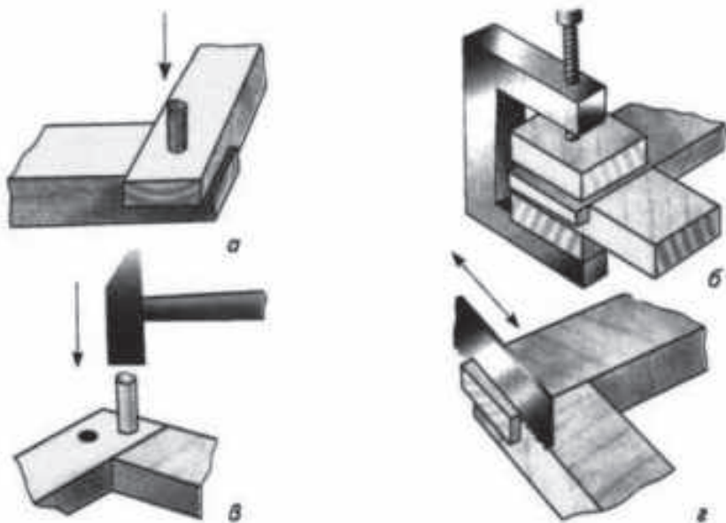
Расми 12. Ширешкунӣ ва коркарди тахтачаҳо: а – маҳкам кардани тахтачаҳо бо меҳи чӯбӣ; б – маҳкам кардани пайвастигиҳои ширешӣ дар гироҳо; в – ҷойгиршавии меҳи чӯбӣ; г – арракунии қадбур.
