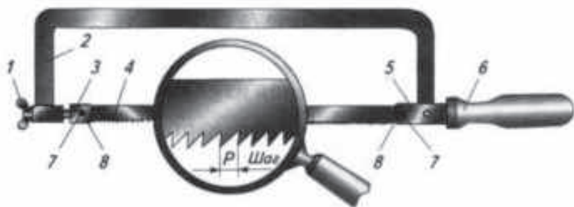
Расми 37. Дастарра: 1 – печ; 2 – чорчӯба; 3 – сараки ҳаракатнок; 4 – тасмаоханги дастарра; 5 – сараки беҳаракат; 6 – думак бо дастак; 7 – пайвандакҳо; 8 – ҷойҳои буридашуда.
