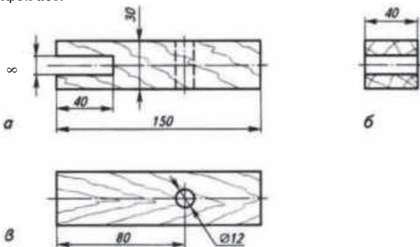
Расми 4. Нақшаи чузъиёти призматикӣ: а – намуди асосӣ, б – намуд аз чап, в – намуд аз боло.
