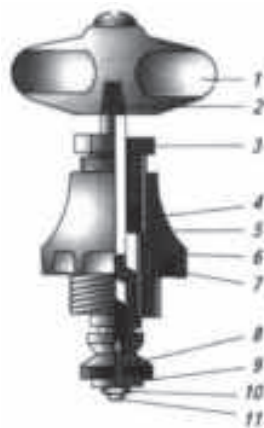
Расми 58. Сохти сараки вентил
