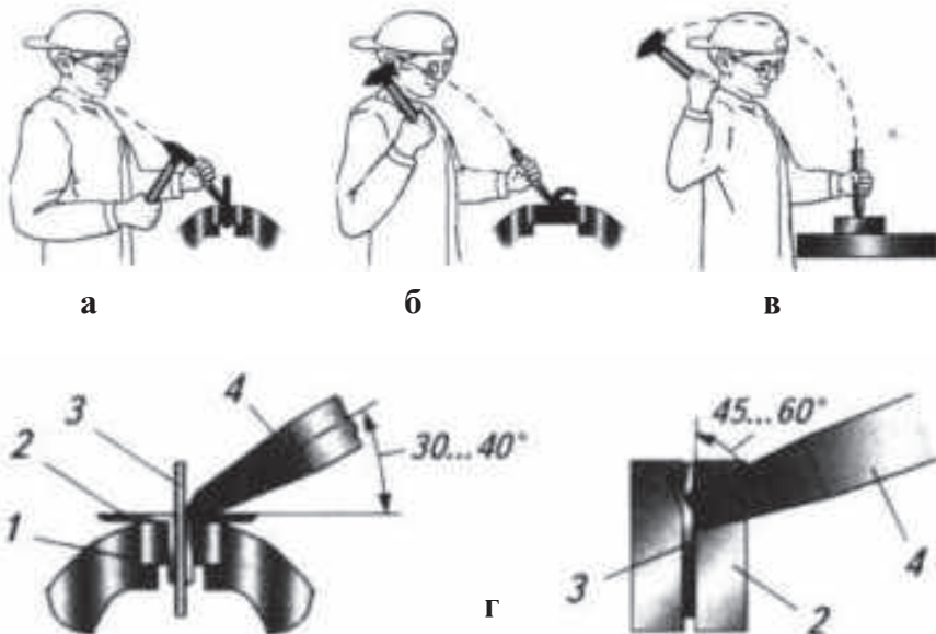
Расми 42. Усули буридани филиз дар гиро: а – зарбаи панчагӣ; б – зарбаи оринҷӣ; в – зарбаи китфӣ; г – ҳолати искана дар вақти буриш: 1 – гиро; 2 – лабакҳо; 3 – масолех; 4 – искана:
