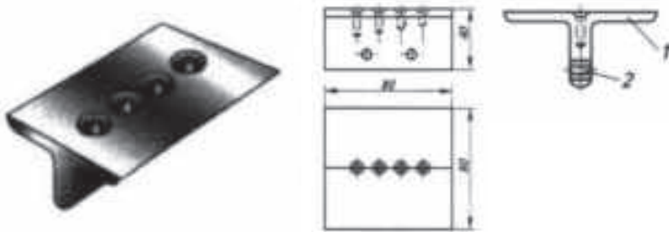
Расми 31. Расми техникӣ (а) ва нақшаи ҷамъшуда (б). Ускуна барои тайёр кардани мехпарчин: 1 – кунҷак; 2 – иштифт.
